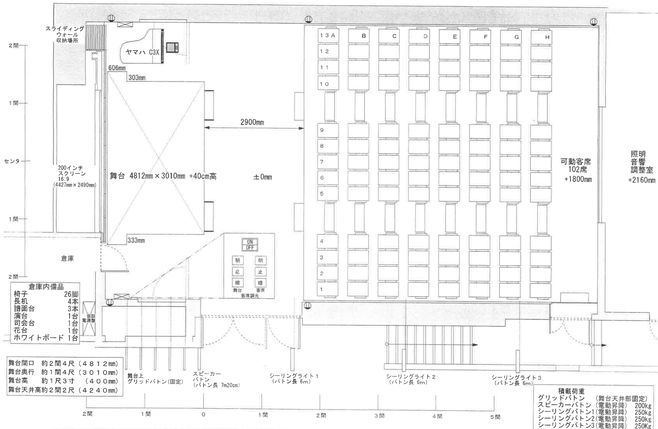
白山市松任学習センター プララ ライブシアター平面図
